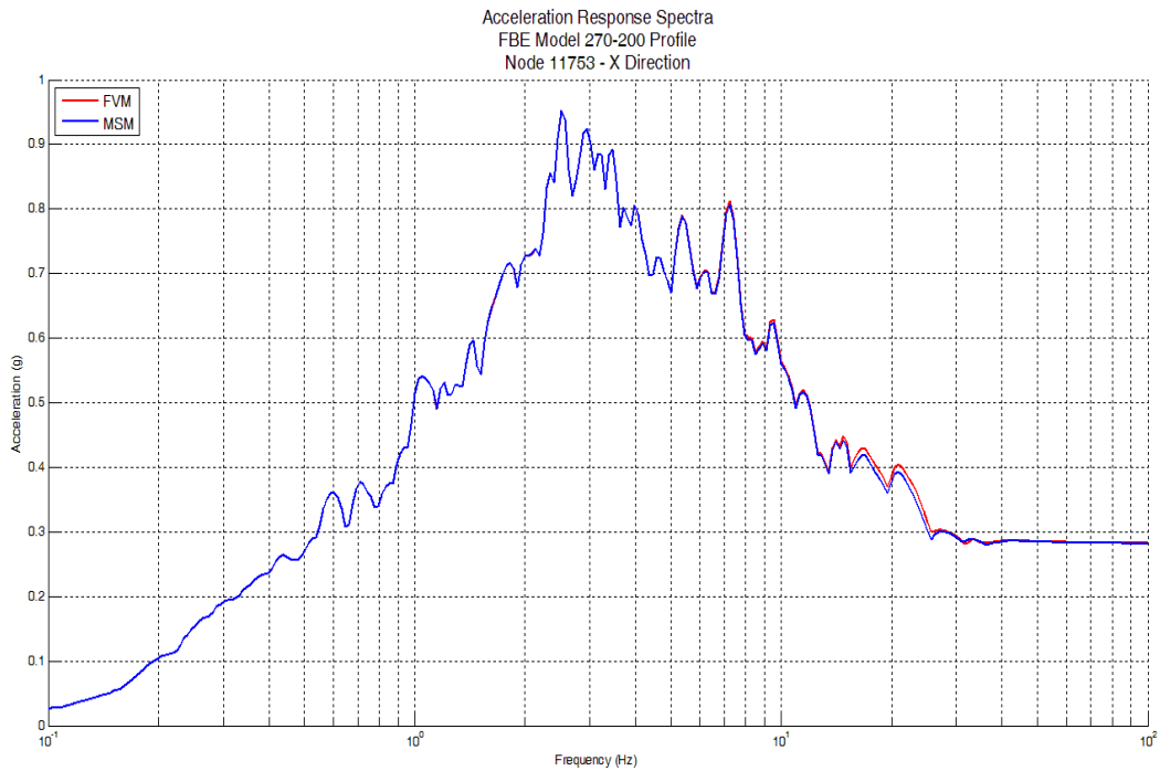
b) 5% Damping ARS
